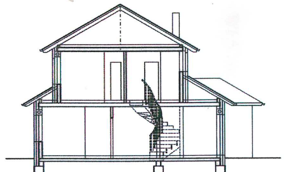
Schnitt Wohnhaus
