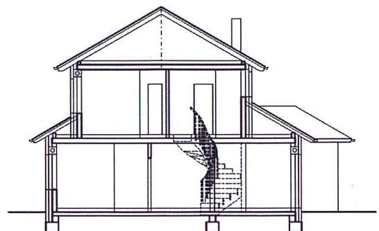
Schnitt Wohnhaus
